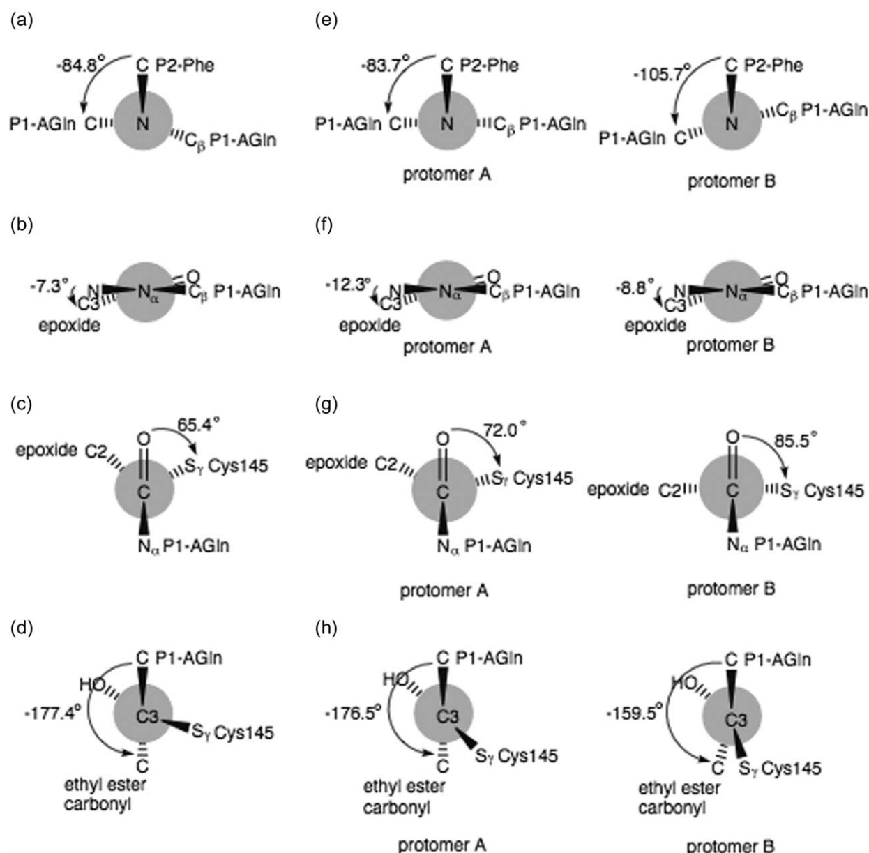
Figure 5. Newman projections. (a) The equivalent to \phi of P1-AGln, C(P2-Phe)-N(P1-AGln)-N \alpha (P1-AGln)-C(P1-AGln), (b) the equivalent to \psi of P1-AGln, N(P1-AGln)-N \alpha (P1-AGln)-C(P1-AGln)-C3(epoxide), (c) the torsion angle O=C(P1-AGln)-C3(epoxide)-S \gamma (Cys145), and (d) the torsion angle C(P1-AGln)-C3(epoxide)-C2(epoxide)-C(ethyl ester carbonyl) of APE in the structure of the SARS-CoV M pro :APE complex. (e) The equivalent to \phi of P1-AGln, C(P2-Phe)-N(P1-AGln)-N \alpha (P1-AGln)-C(P1-AGln), (f) the equivalent to \psi of P1-AGln, N(P1-AGln)-N \alpha (P1-AGln)-C(P1-AGln)-C3(epoxide), (g) the torsion angles O=C(P1-AGln)-C3(epoxide)-S \gamma (Cys145) and (h) the torsion angle C(P1-AGln)-C3(epoxide)-C2(epoxide)-C(ethyl ester carbonyl) of APE in protomers A and B of the M pro +A(-1) :APE complex.
